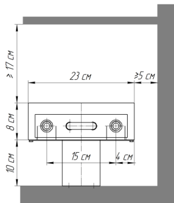
Исполнение "нв" (нерегулируемая высота)
