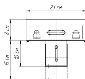
Исполнение "рв" (регулируемая высота)
