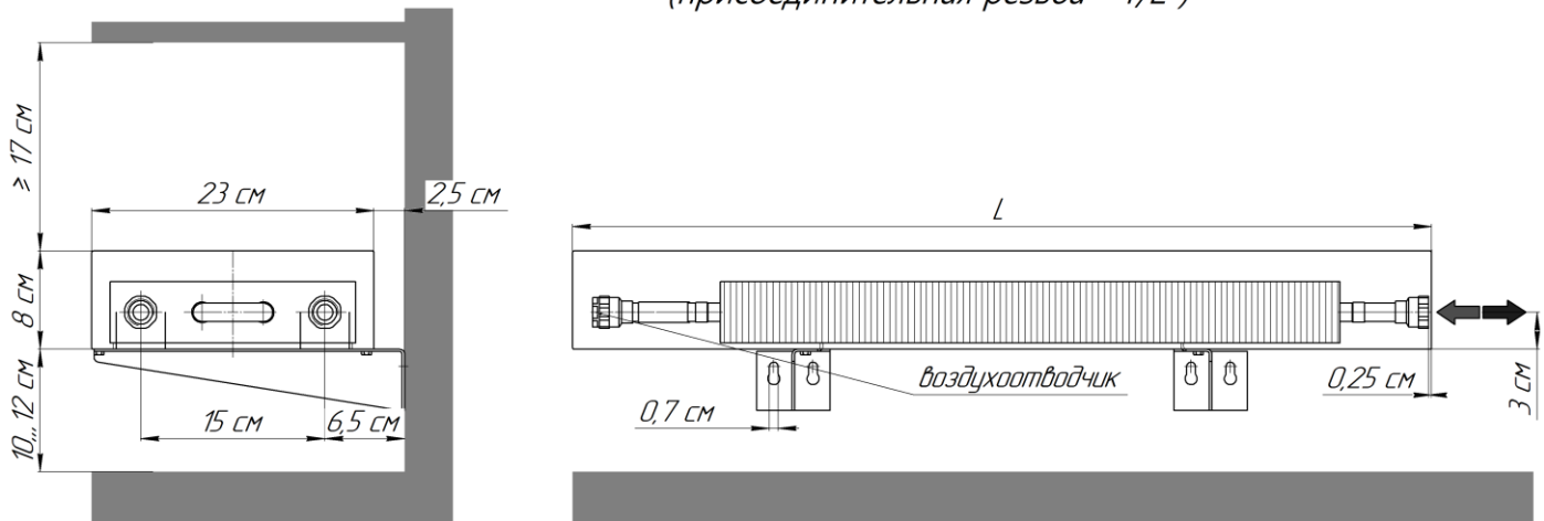
Настенный конвектор "Элегант - мини 230х80-2то бок Стен прав" с правосторонним боковым присоединением (левостороннее - зеркально) (присоединительная резьба - 1/2")
