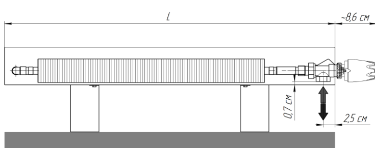
Вид для исполнения "нв" (нерегулируемая высота)
