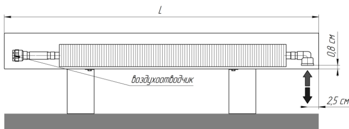
Вид для исполнения "нв" (нерегулируемая высота)
